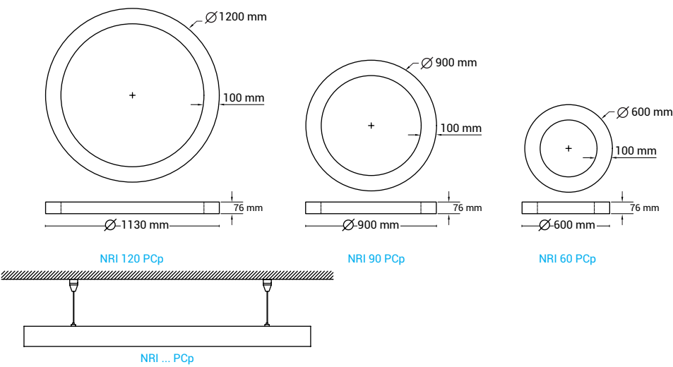
LED(SMD) Module
